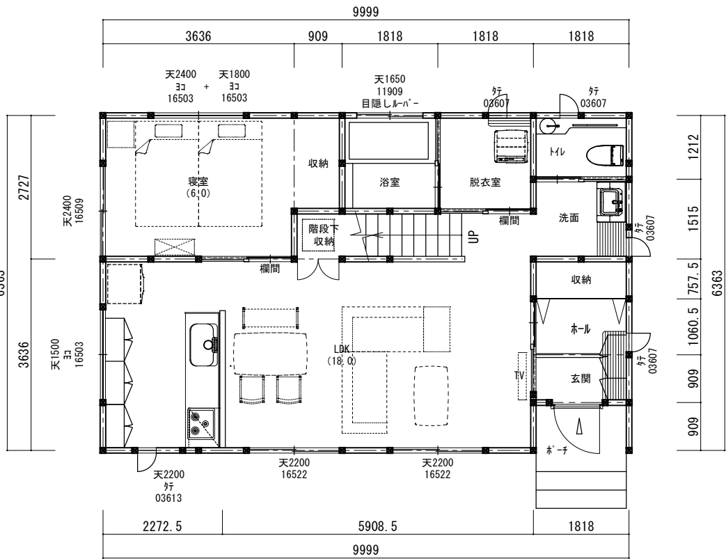
1 階平面図
