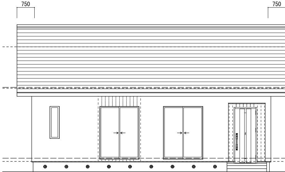
側立面図
