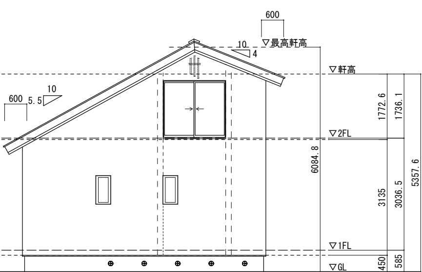
側立面図
