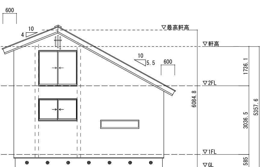
側立面図
