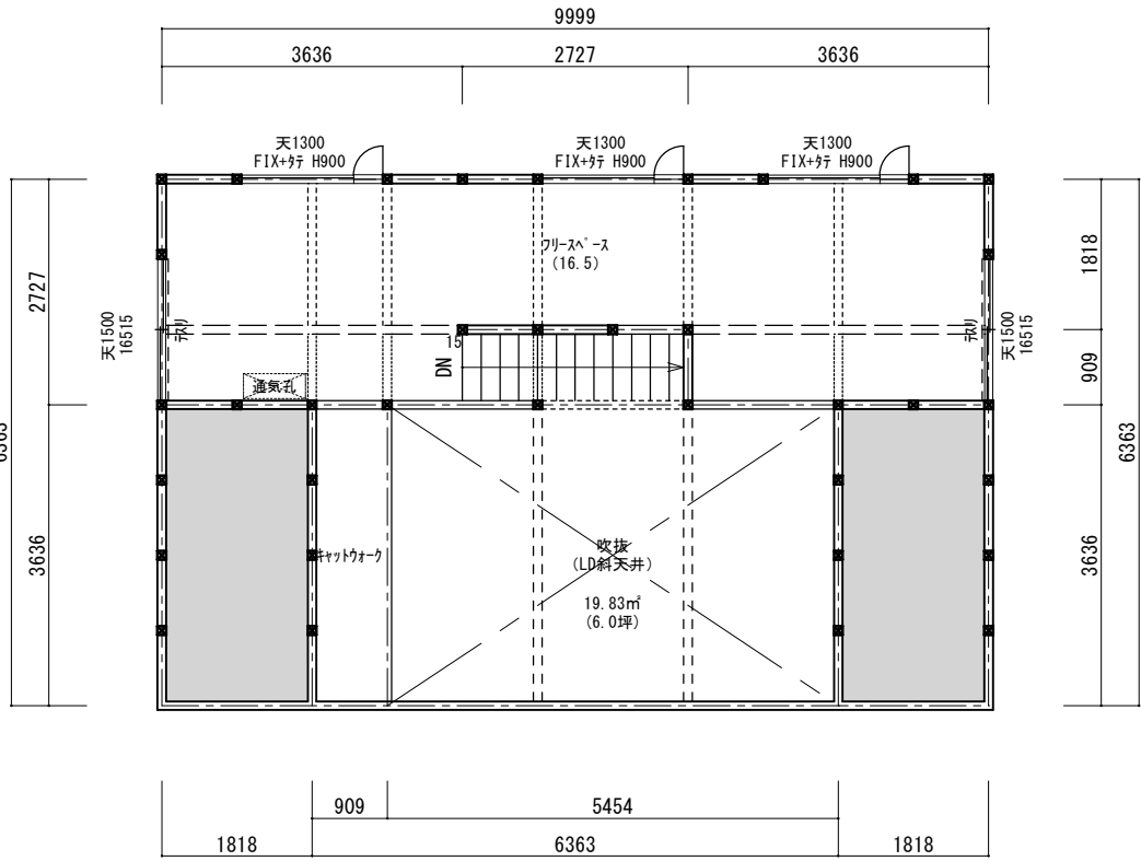
2 階平面図
