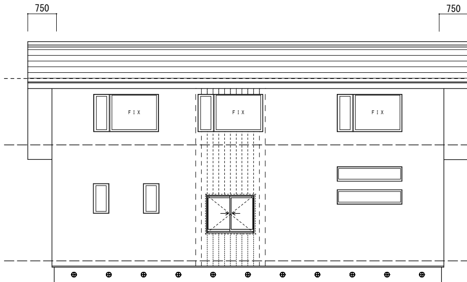
側立面図
