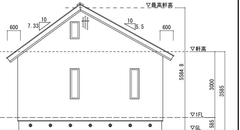
側立面図
