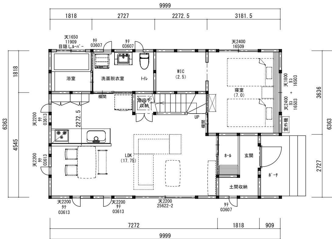
1階平面図
